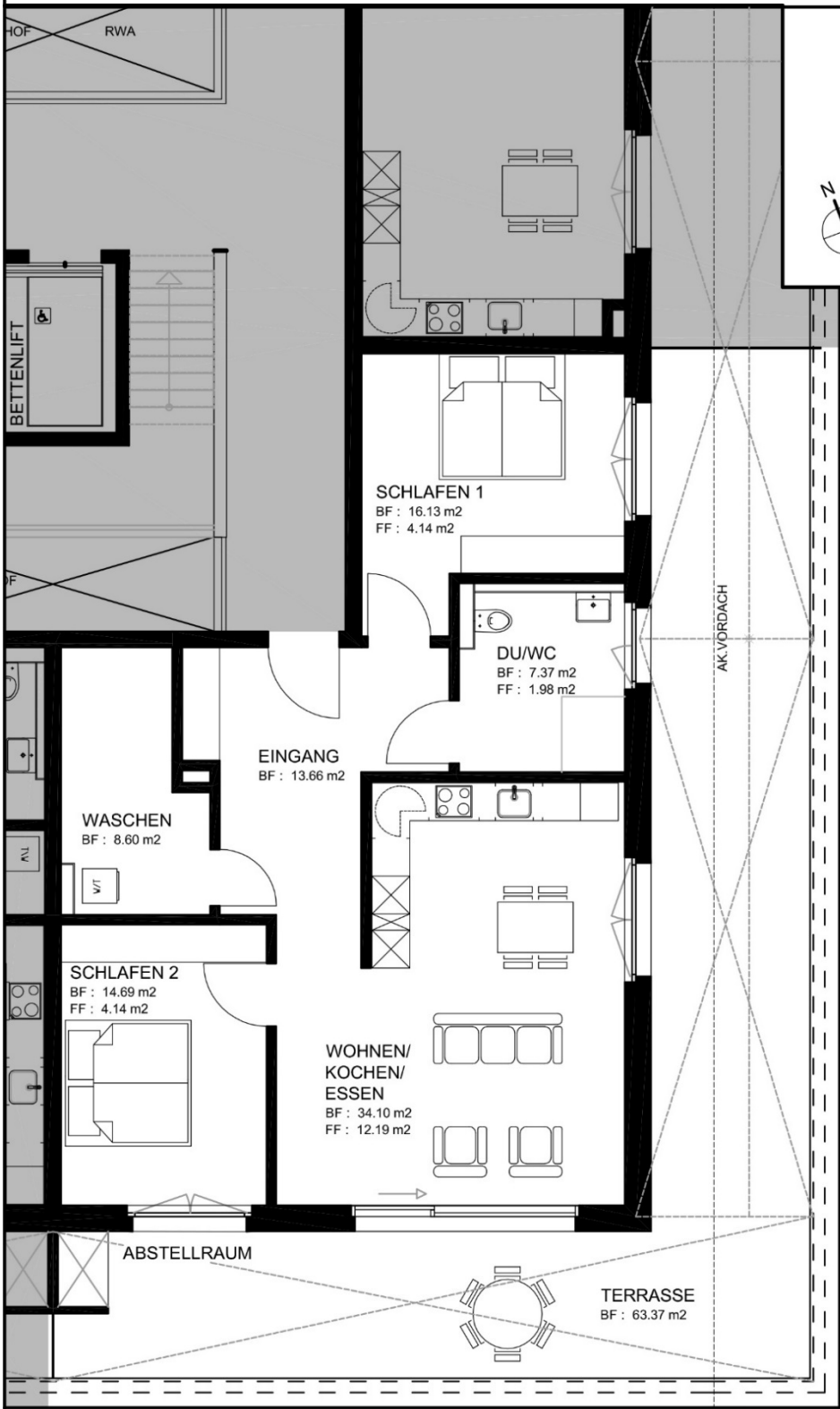
TYP 3.2 ATTIKA 3.5 ZI. WHG. NETTOFLÄCHE 94.5 M 2
